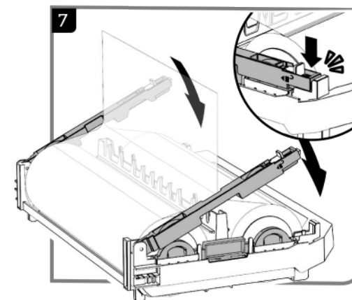
7. アームバーを元の位置に戻しロックされるまで押し下げる
