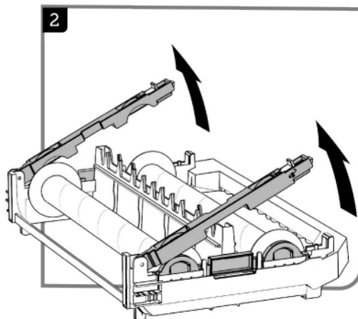
2. ロックをスライドしたままアームバーを持ち上げ180度回転させる
