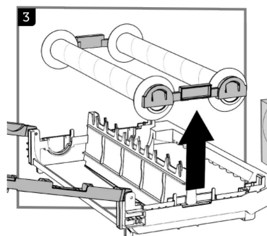
3. 空になったロールフィルムを取り外す
