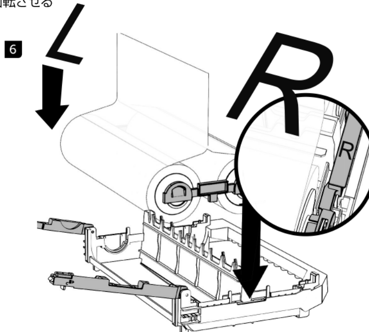
6. カートリッジ外枠とロールフィルム左右を合わせてセットする
