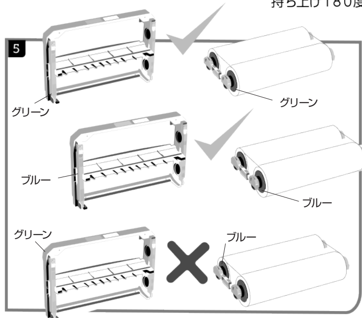
5. カートリッジ外枠とロールフィルムの組み合わせに注意 同じ色のカートリッジ外枠とロールフィルムしか使用できません
